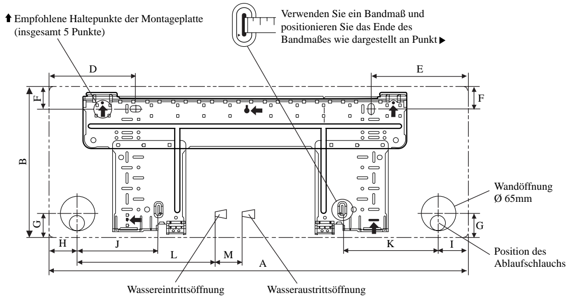
MONTAGEPLATTE FWT02/03/04
