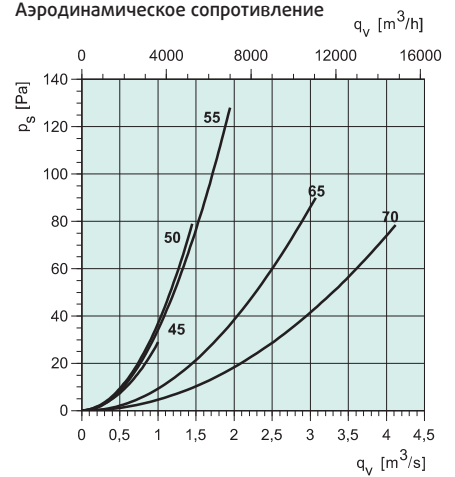
Аэродинамическое сопротивление
