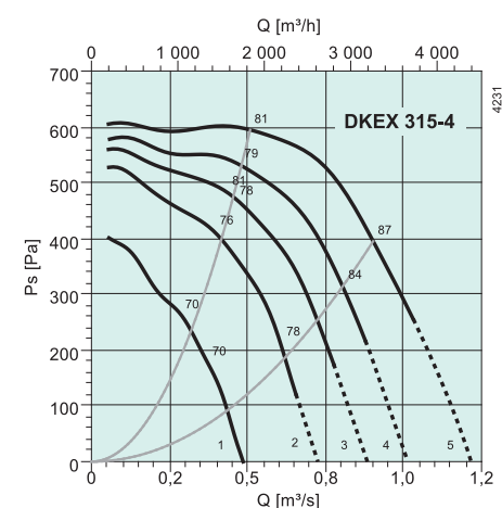
Мин. статическое давление 250 Па
