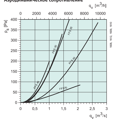
Аэродинамическое сопротивление
