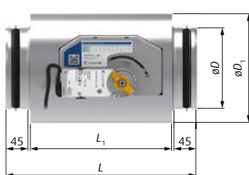
Рис. 3 Размеры NOTUS-RI-M1
