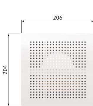
Рисунок 1. BOR-S, типоразмеры: BOR-S-100: \varnothing = 99 мм BOR-S-125: \varnothing = 124 мм
