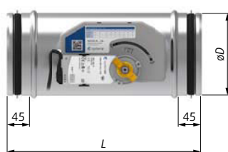
Рис. 2 Размеры NOTUS-R-M1
