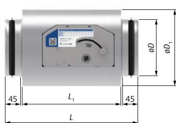
Рис. 3 Размеры NOTUS-RI-M0
