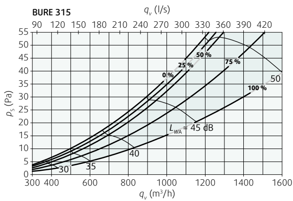
Диаграмма 2а: Падение давления и уровень звуковой мощности. (Все типы диффузоров BURE).
