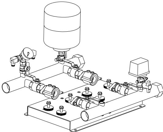
Рис. 6 Рама-основание, коллекторы и клапаны
