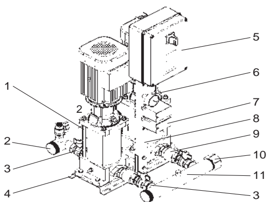
Рис. 1 Установка повышения давления Hydro Multi-S
