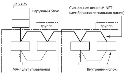
Система с МА-пультом управления
