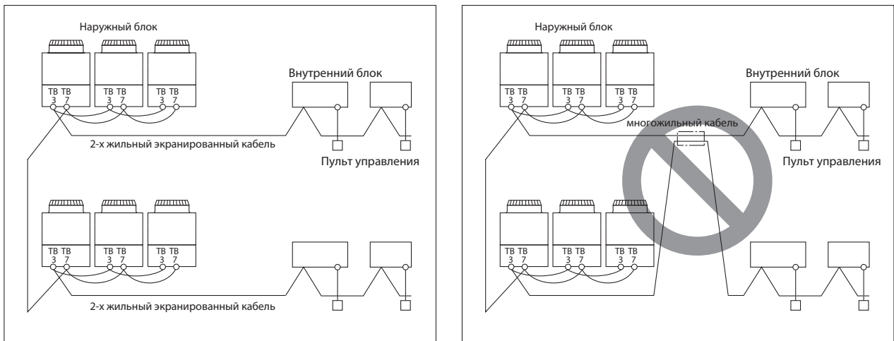
ТВ3: клеммная колодка межблочной сигнальной линии, ТВ7: клеммная колодка централизованного управления.
