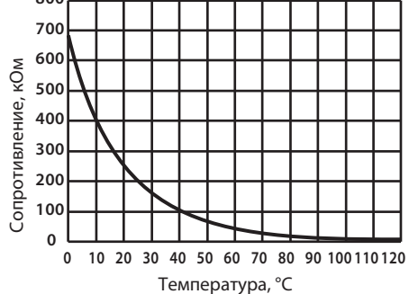
Термистор температуры нагнетания (RT62)
