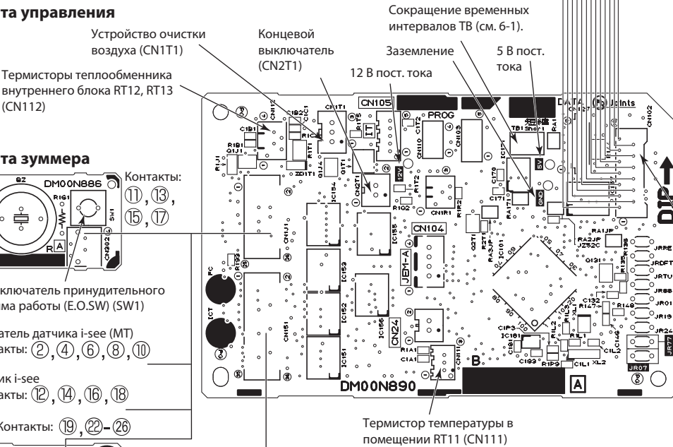
Разъем для платы питания внутреннего блока (CN102)
