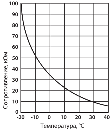
Термистор оттаивания (RT61) Термистор наружной температуры (RT65) Термистор теплообменника наружного блока (RT68)
