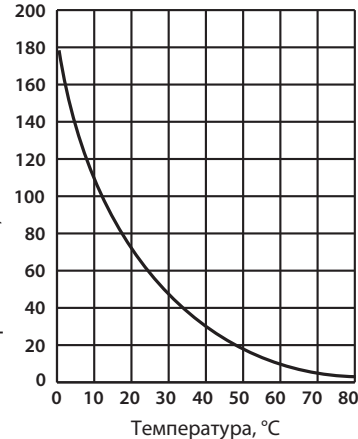
Термистор температуры тепловода (RT64)
