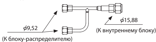
② Объединитель (газ)
