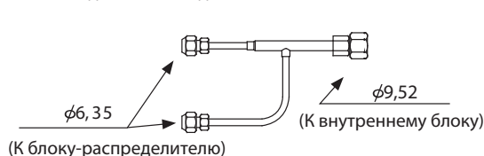
③ Объединитель (жидкость)
