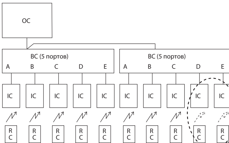
в) два 5-ти портовых BC (максимум 8 внутренних блоков)
