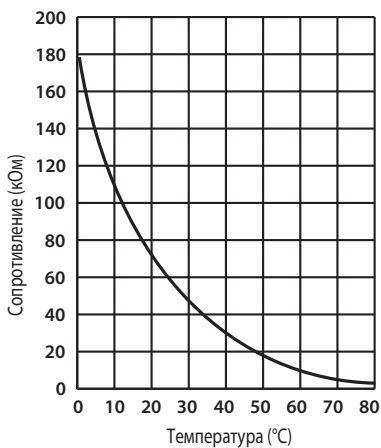
Термистор температуры тепловода (RT64)
