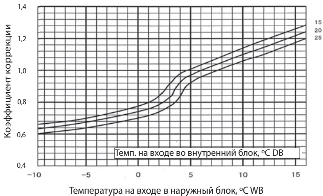
Рис. 4-3. Теплопроизводительность
