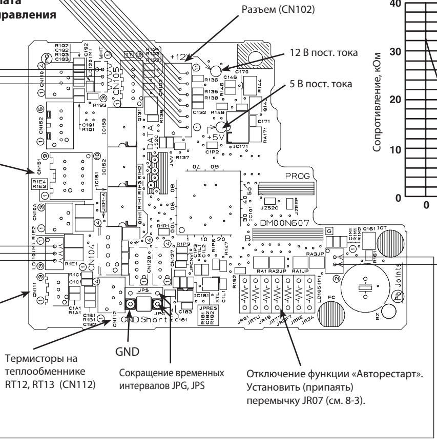
Термистор комнатной температуры RT11 Термисторы на теплообменнике (RT12, RT13)
